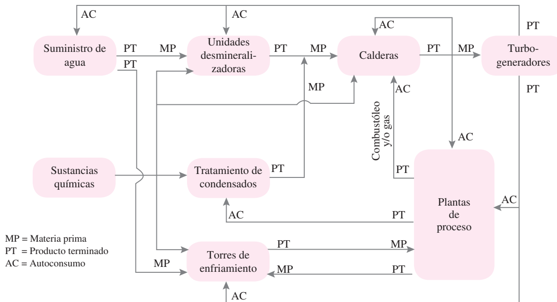
♥ Ilustración 5.7 Diagrama general de proceso (cadena de producción).
