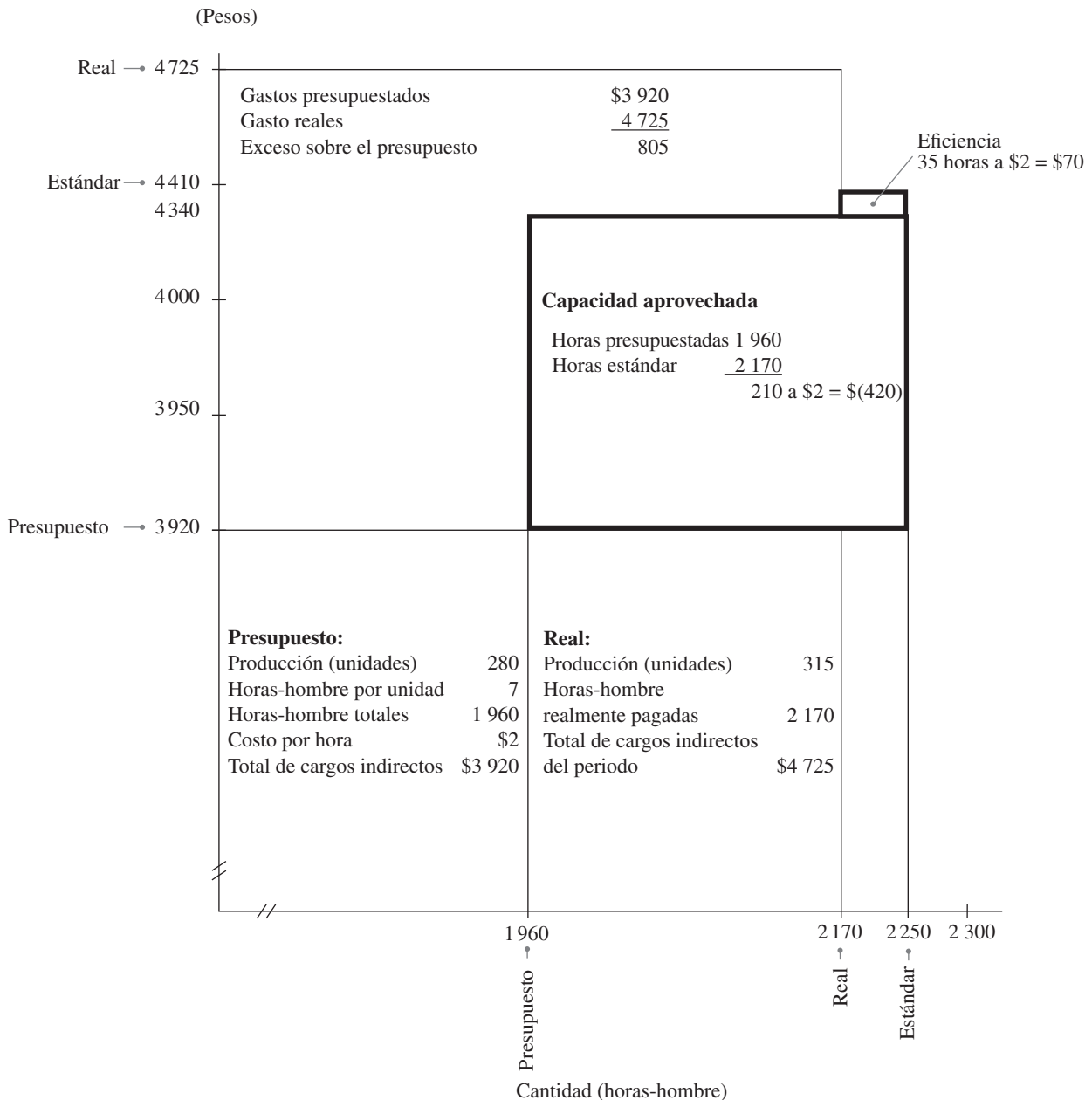
♥ Ilustración 8.12 Análisis gráfico de variaciones en cargos indirectos.
